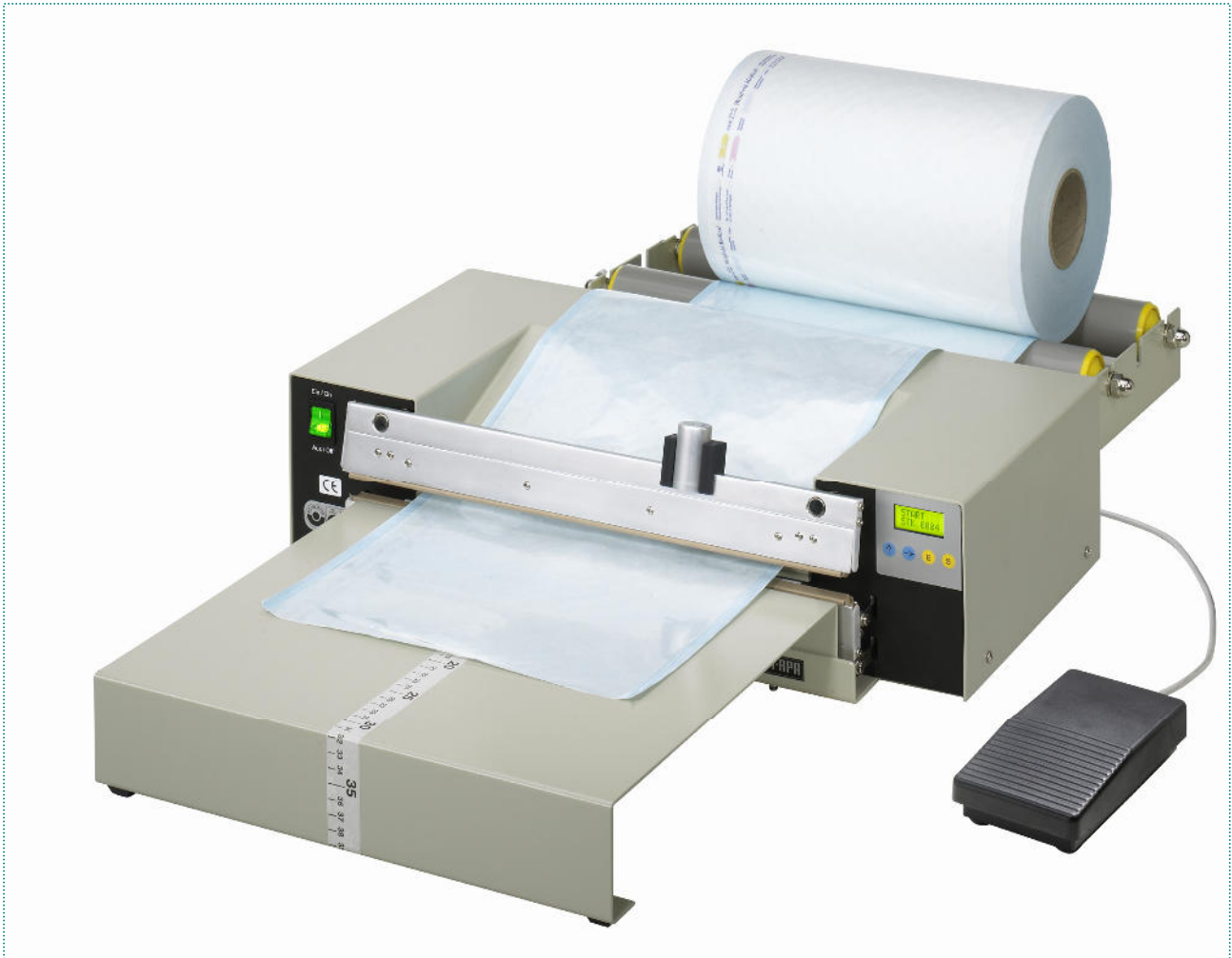
polystar® 418 M-RPA mit Schneidvorrichtung (SV), Anstecktisch und Folienabroller
