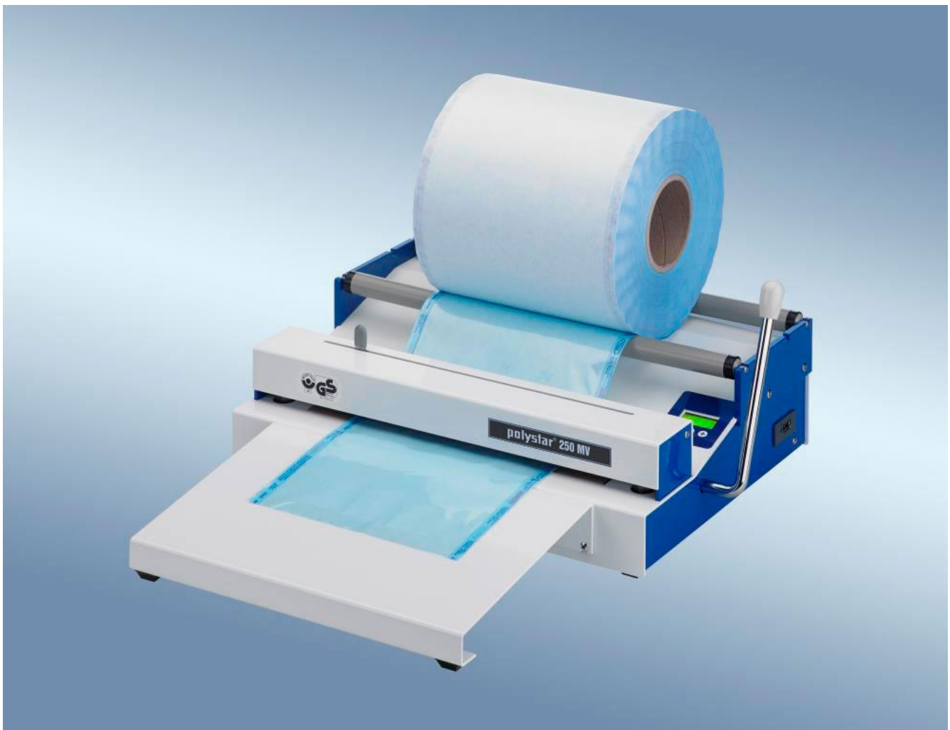
polystar® 250 MV mit Schneidvorrichtung, Anstecktisch und Folienabroller
